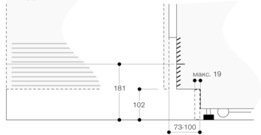
Цоколь. Детали
